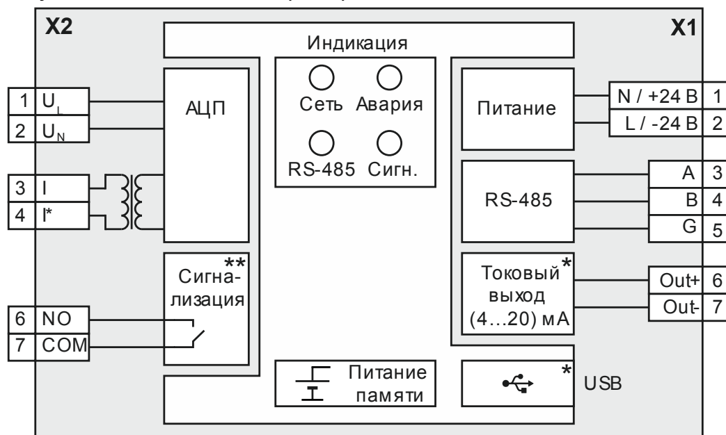
Рисунок 2 – Функциональная схема преобразователя НПСИ-500-МС1.X-X-X-M0, гальваническая изоляция
